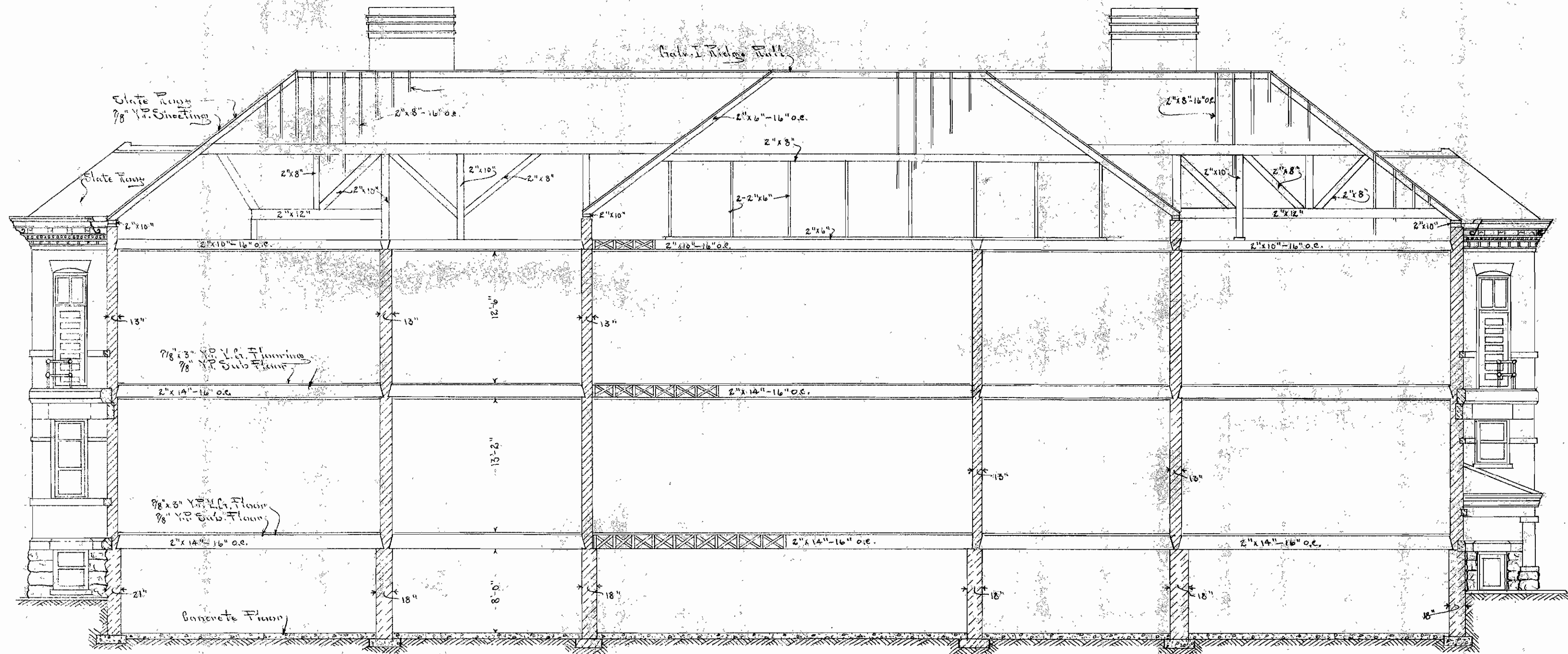
LONGITUDINAL - SECTION
