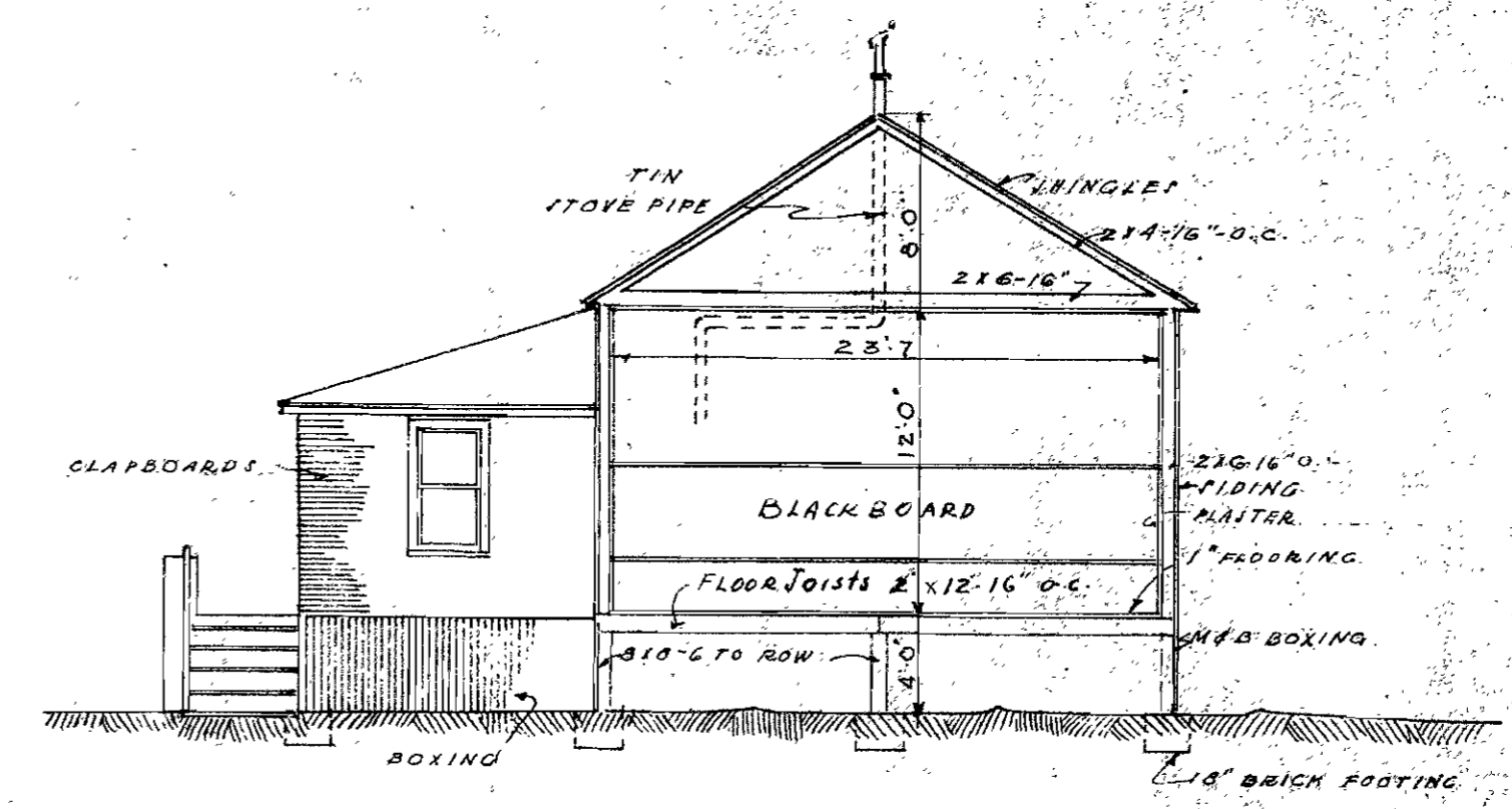
· SECTION ·
