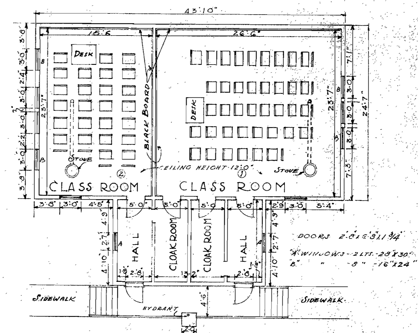
· FLOOR · PLAN · SCALE 0 2 4 6 8 12
