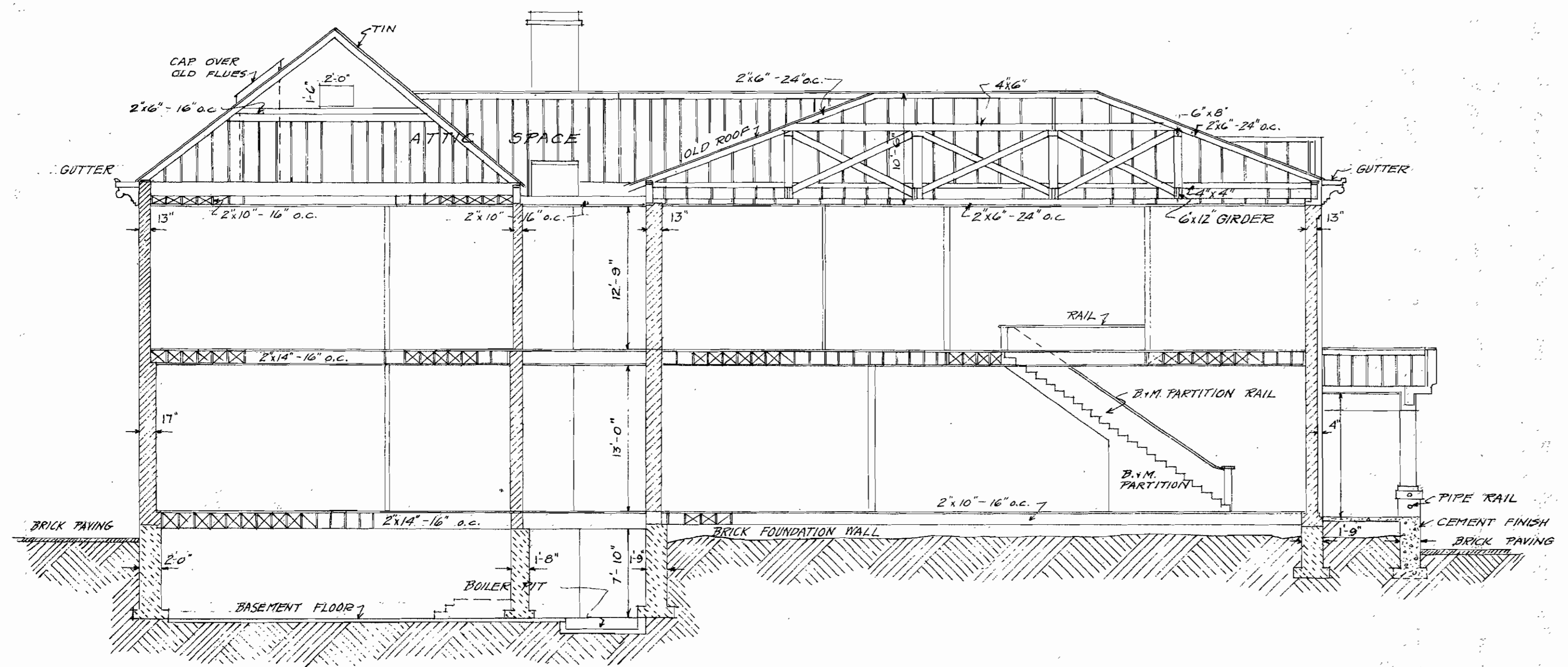
LONGITUDINAL SECTION SCALE 0 2 4 6 8 12
