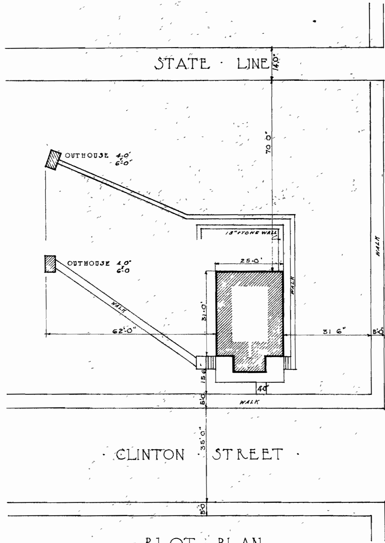
· PLOT PLAN · SCALE 0 5 10 15 20 30
