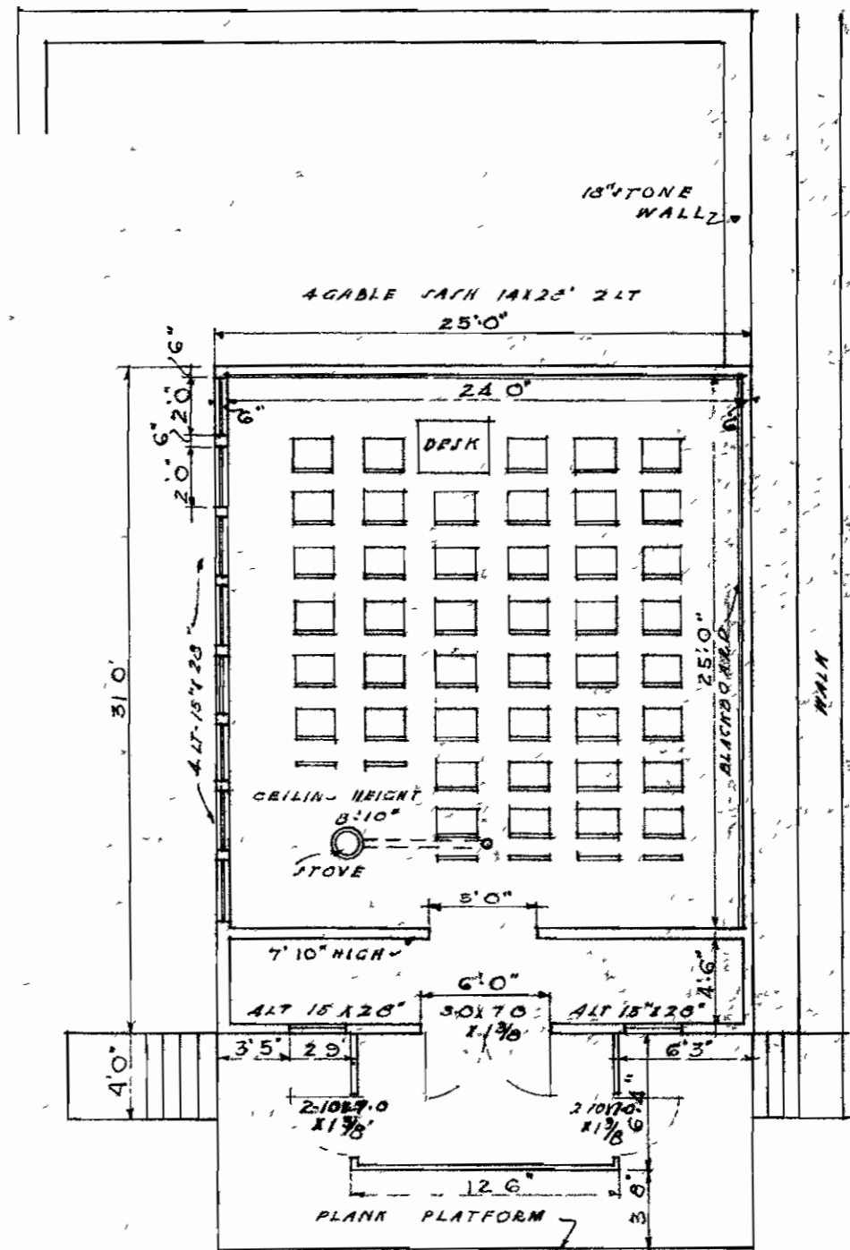
· FLOOR PLAN ·
