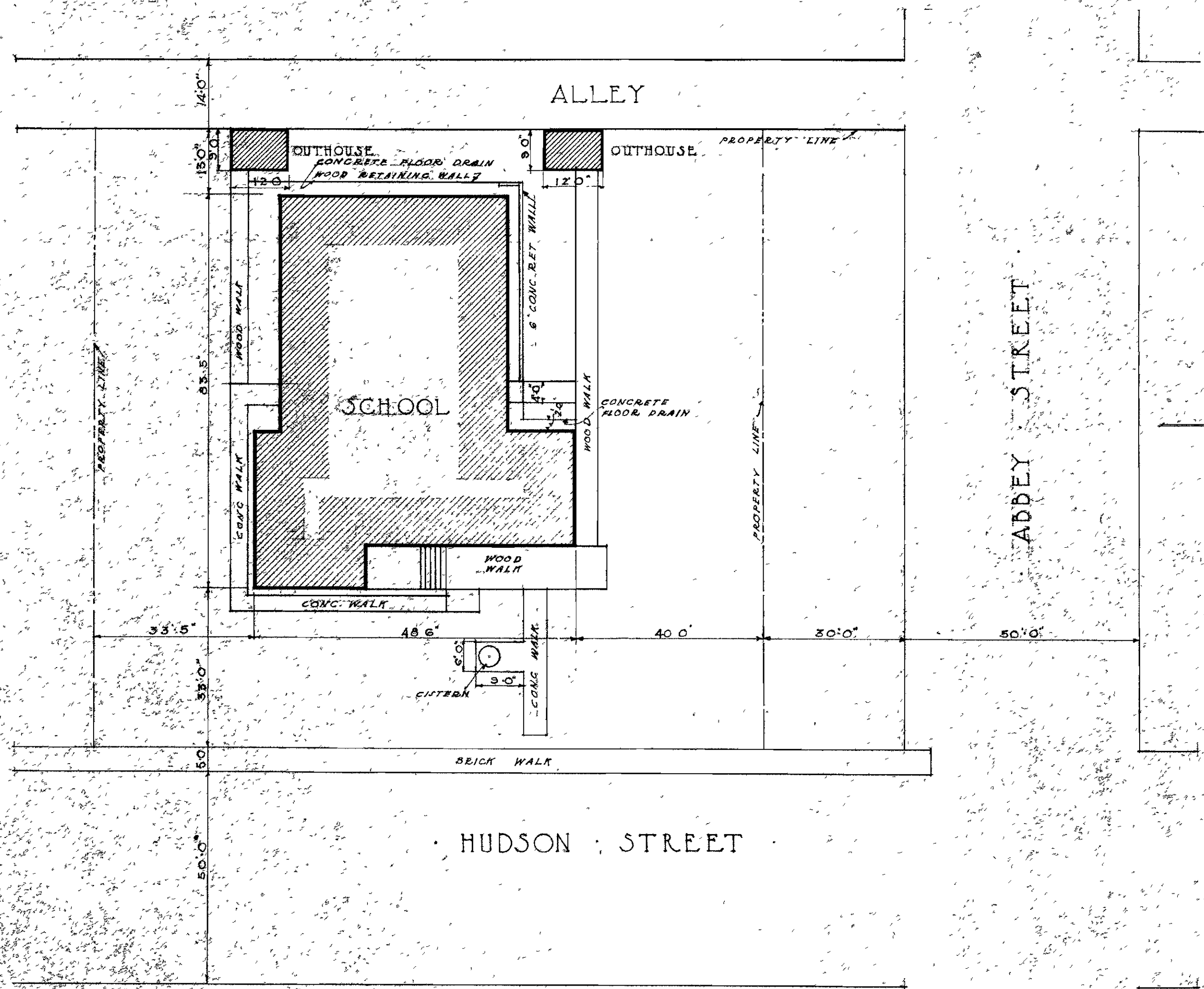
· PLOT PLAN · SCALE 0 5 10 15 20 30 · GREY STONE · SCHOOL ·
