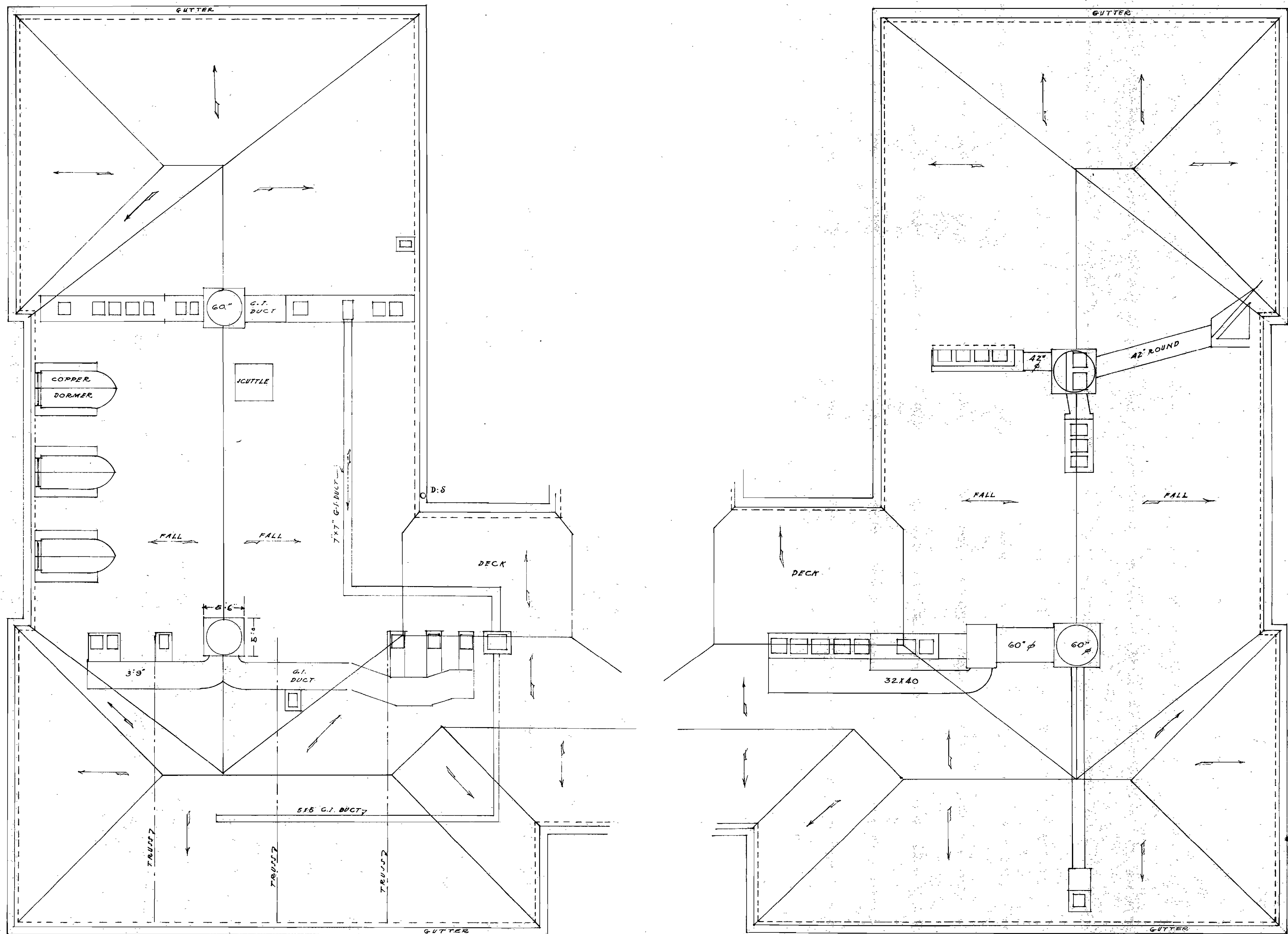
· ATTIC · AND · ROOF · PLAN ·
