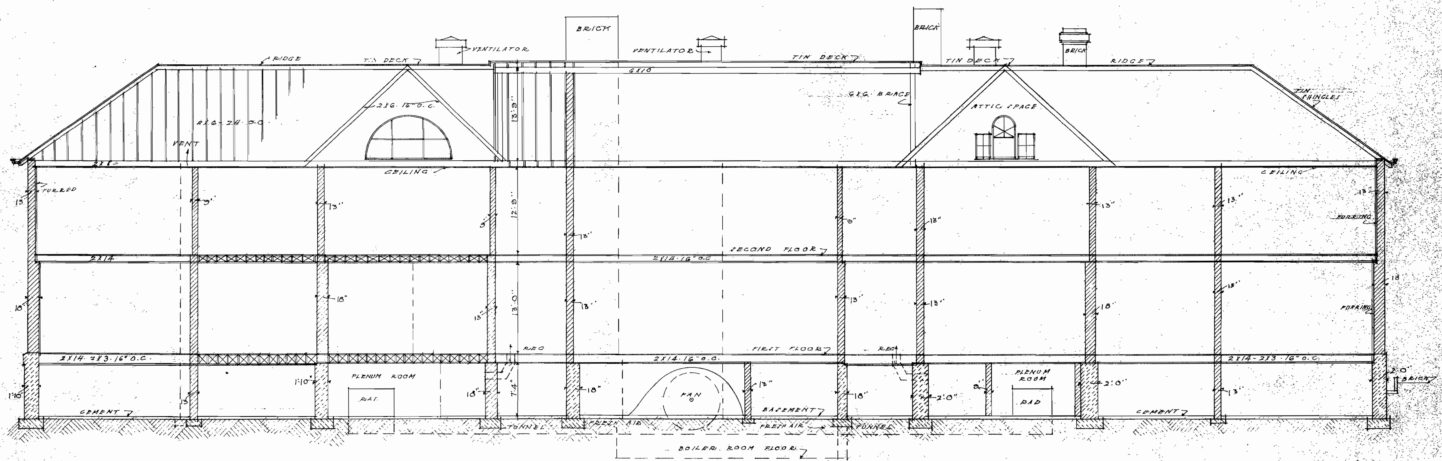
LONGITUDINAL SECTION SCALE 0 2 4 6 8 12
