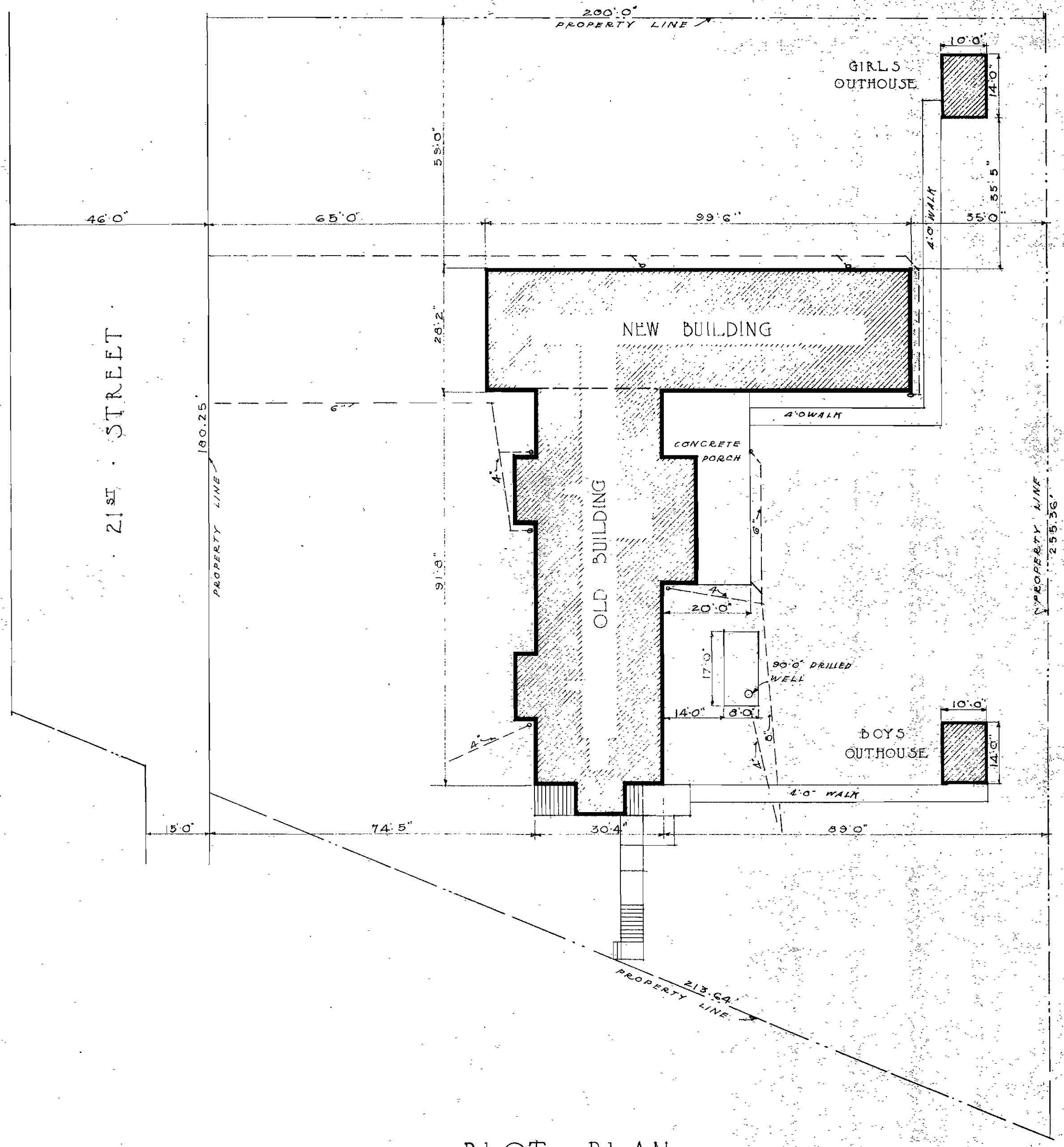
· PLOT · PLAN · SCALE 0 5 10 15 20 30
